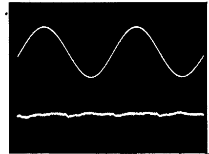
Vervorming (TDH) eindversterker 1 kHz - 40 W - 0,0036%
