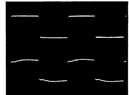
Blokgolf van de Luxman 308. boven in 8Ω, onder in Quad ESL, beide 10 kHz
